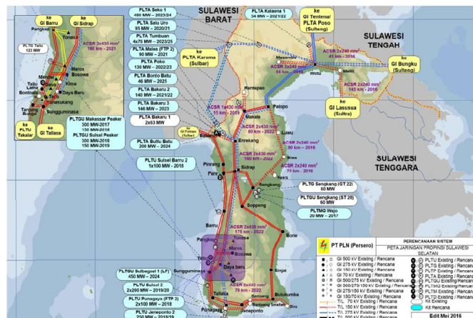
Gambar 1. Peta Jaringan Ketenagalistrikan Provinsi Sulawesi Selatan [1]
