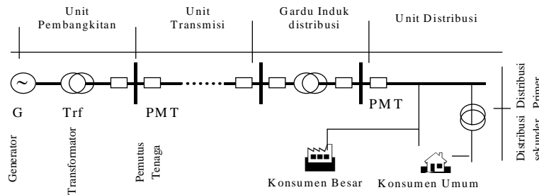
Gambar 3. Diagram segaris suatu sistem sederhana
